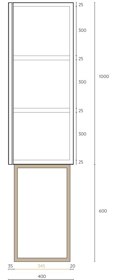
vista in sezione – section view
