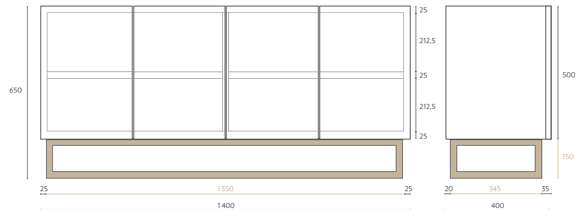
vista di fronte – front view
